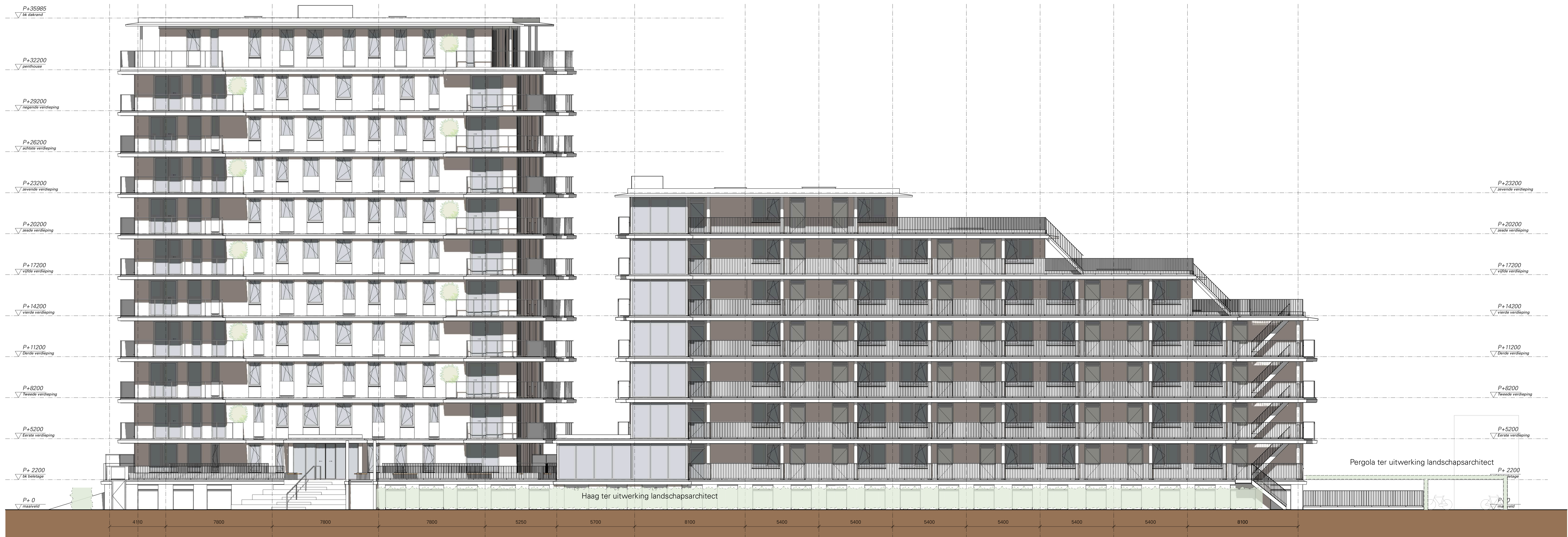
Gevelaanzicht Noord Schaal: 1:100
